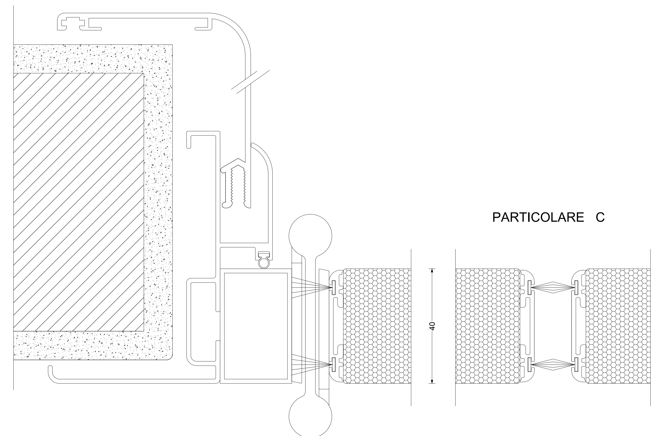
PARTICOLARE B
