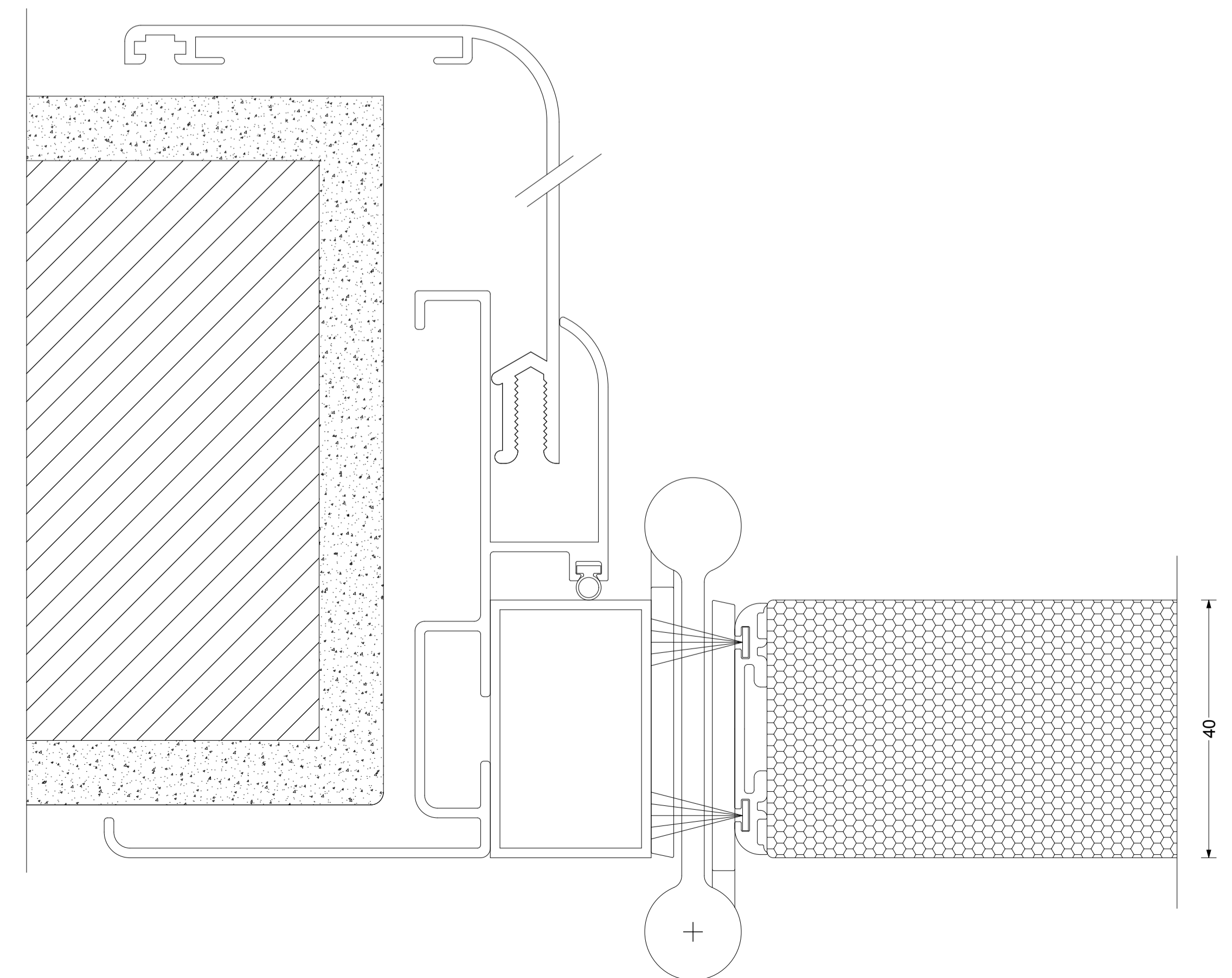
PARTICOLARE B
