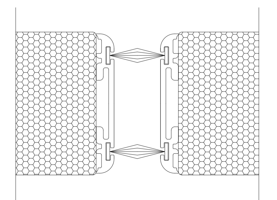
PARTICOLARE C
