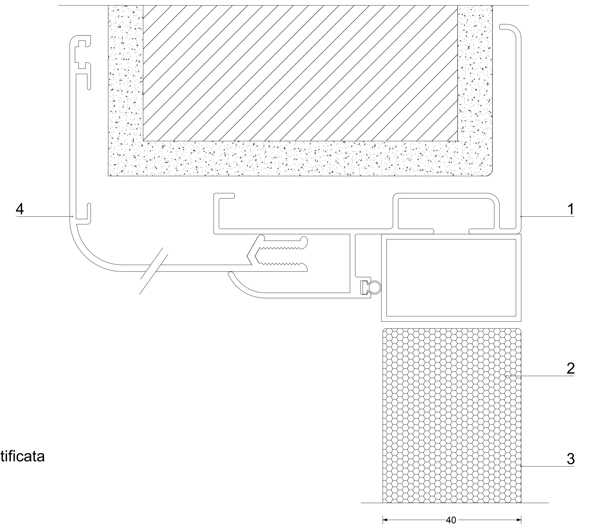
PARTICOLARE A
