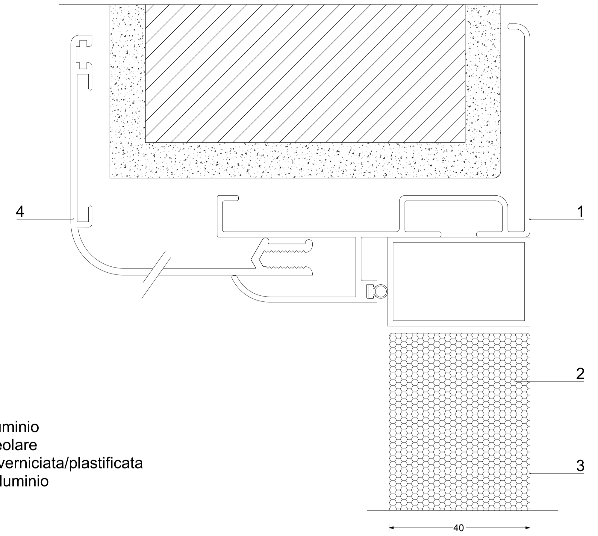
PARTICOLARE A
